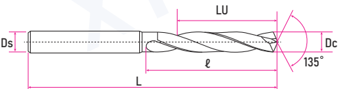
最大推荐钻深 LU=ℓ-1.5D
